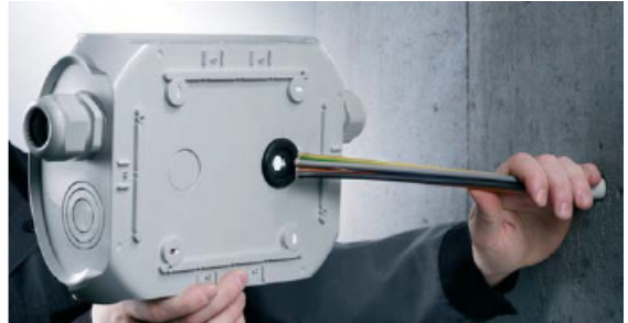
Kabelgenomföring i botten vis ett elastiskt membran.
